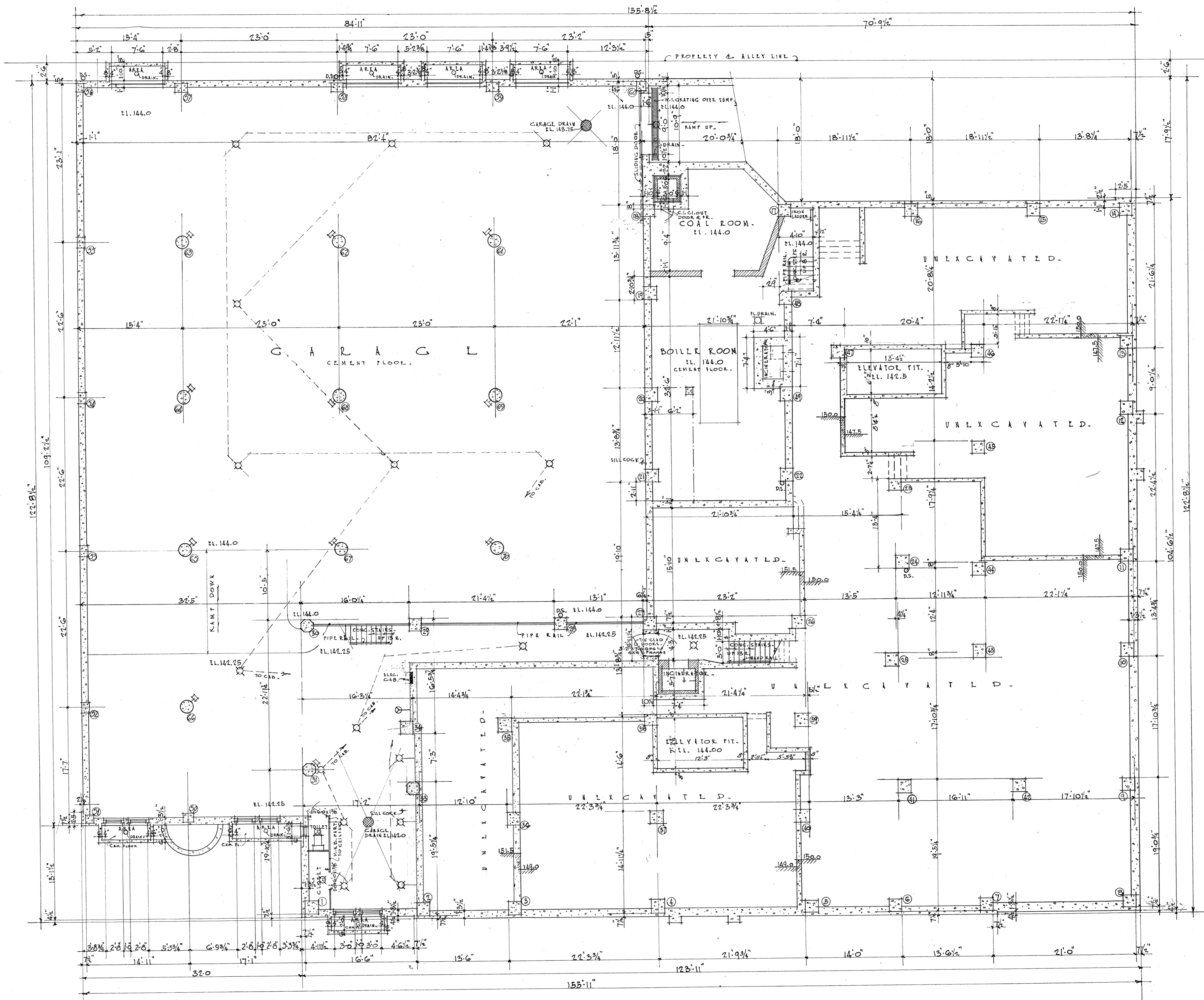
· BASEMENT · PLAN · SCALE: 1/8" = 1'-0"
